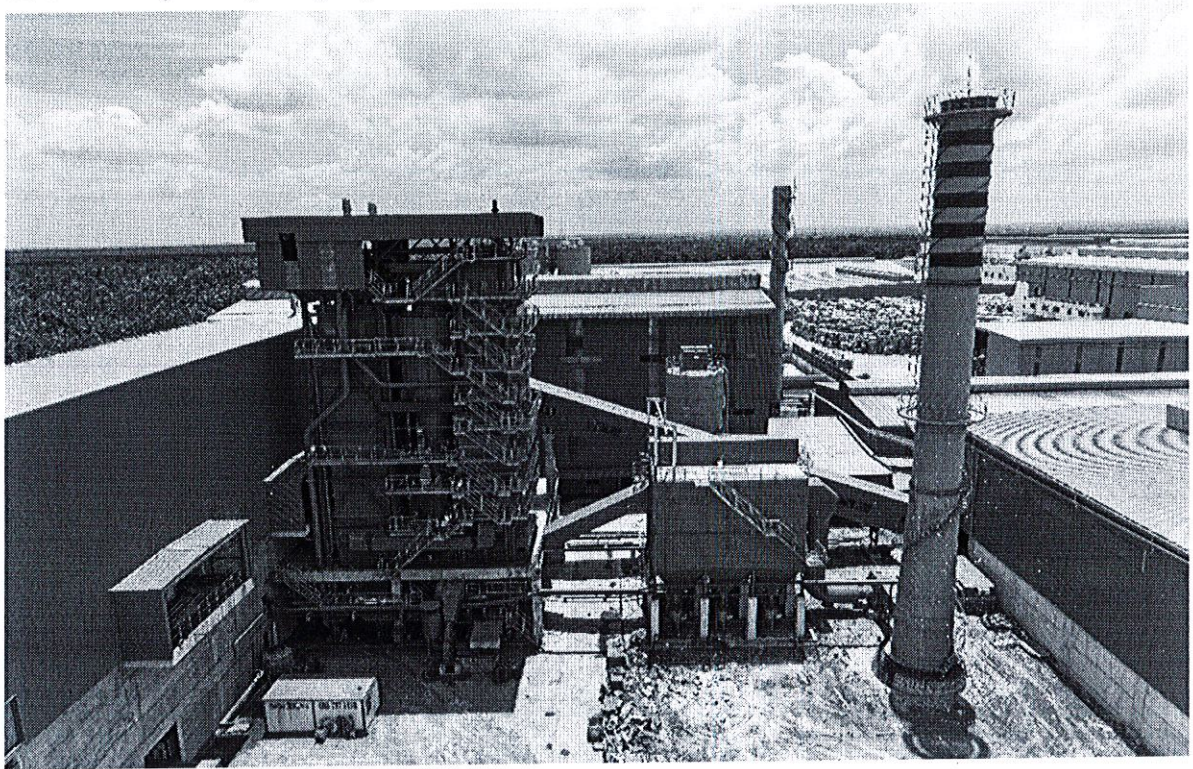
Hình ảnh hệ thống xử lý bụi và khí thải lò hơi
